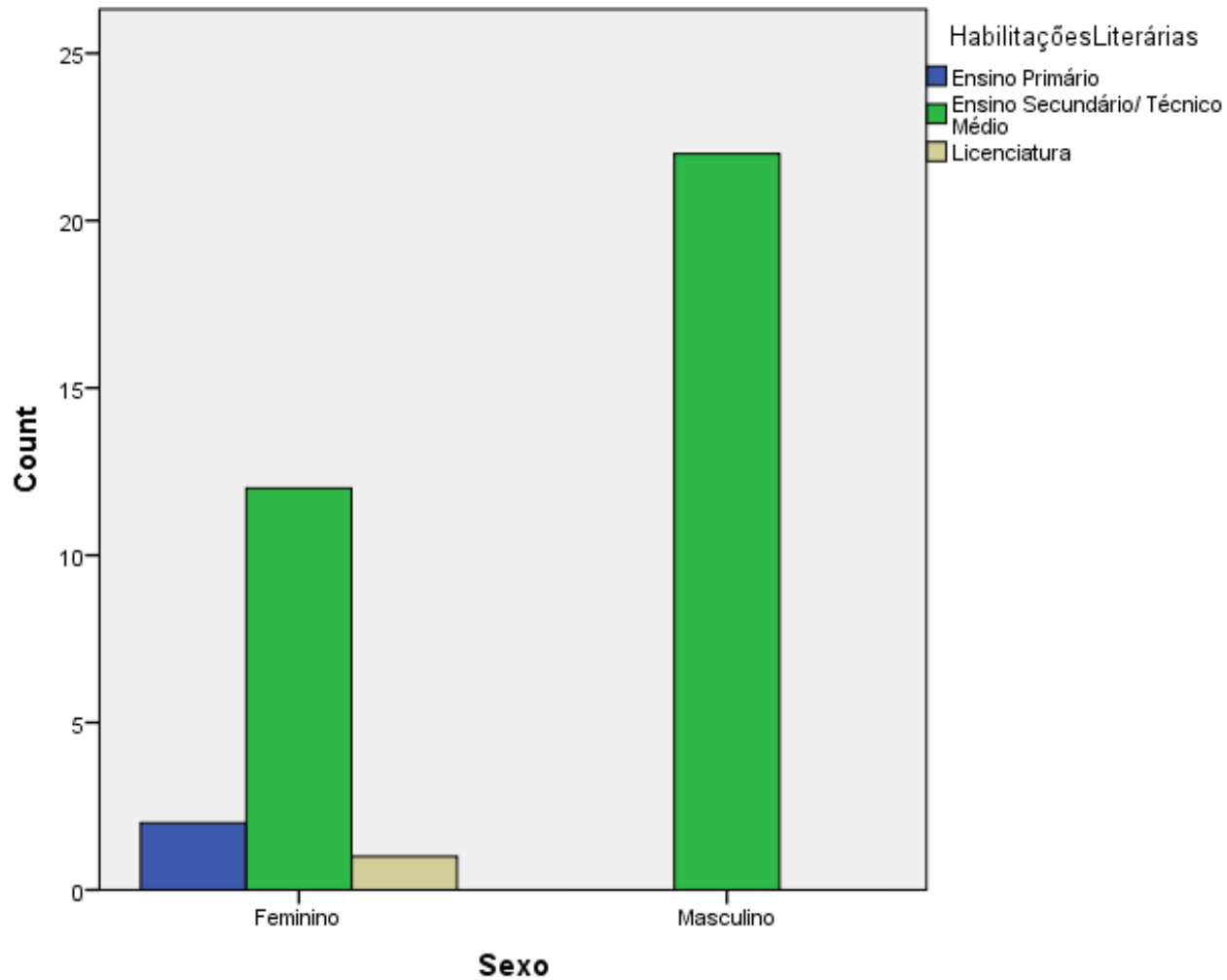
Gráfico 2: Relação entre o Sexo e as Habilitações Lit.
