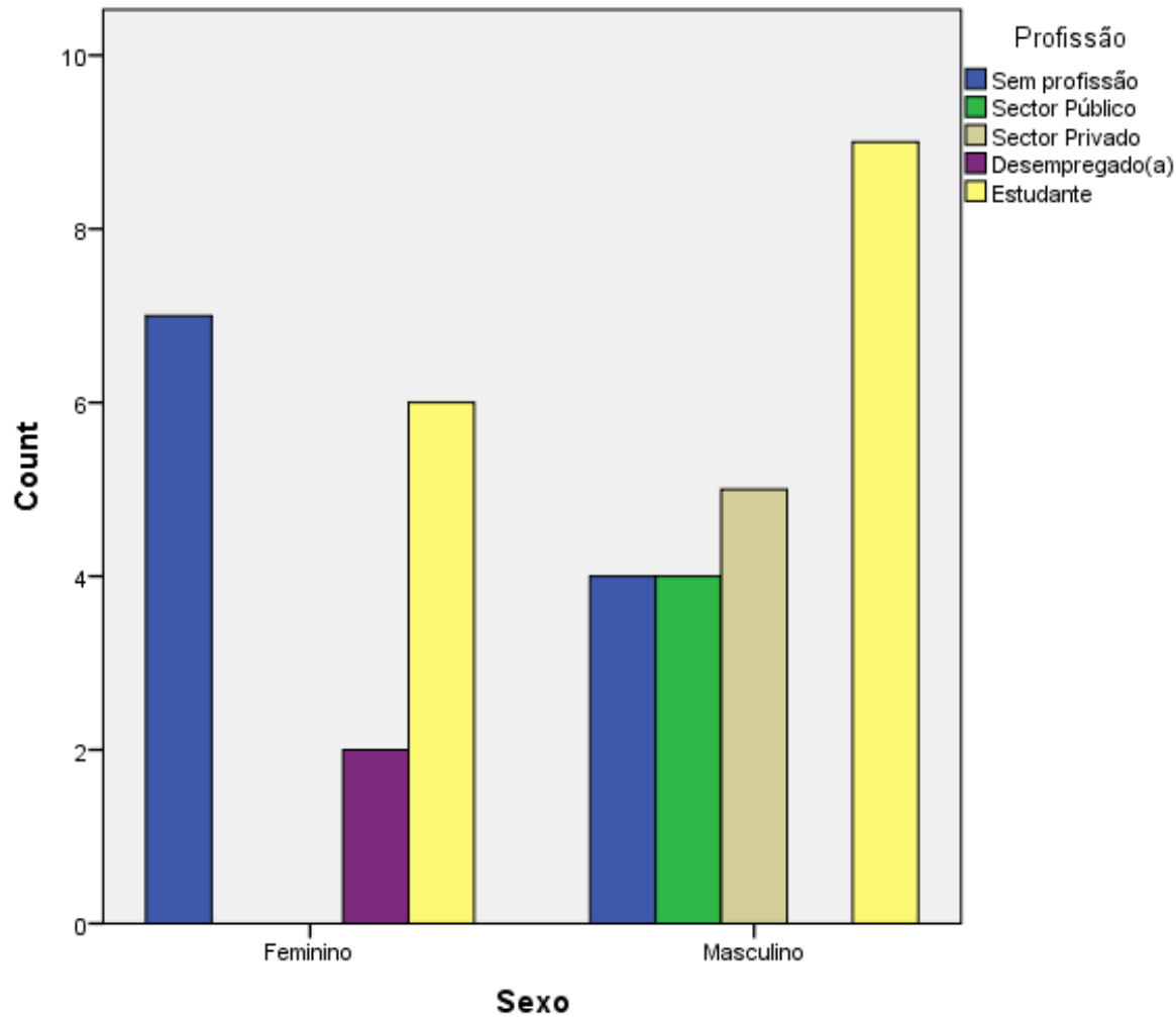
Gráfico 3: Relação entre o Sexo e Profissão.
