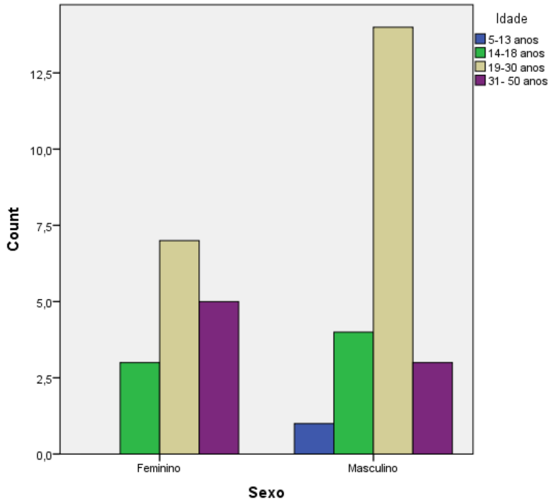
Gráfico 1: Relação entre o Sexo e a Idade.
