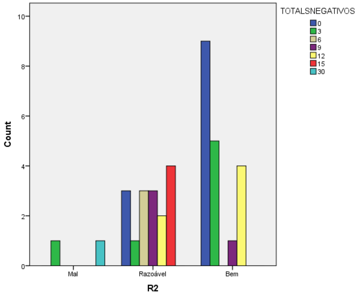
Gráfico 6: Relação entre R2 e o TotalS negativos.
