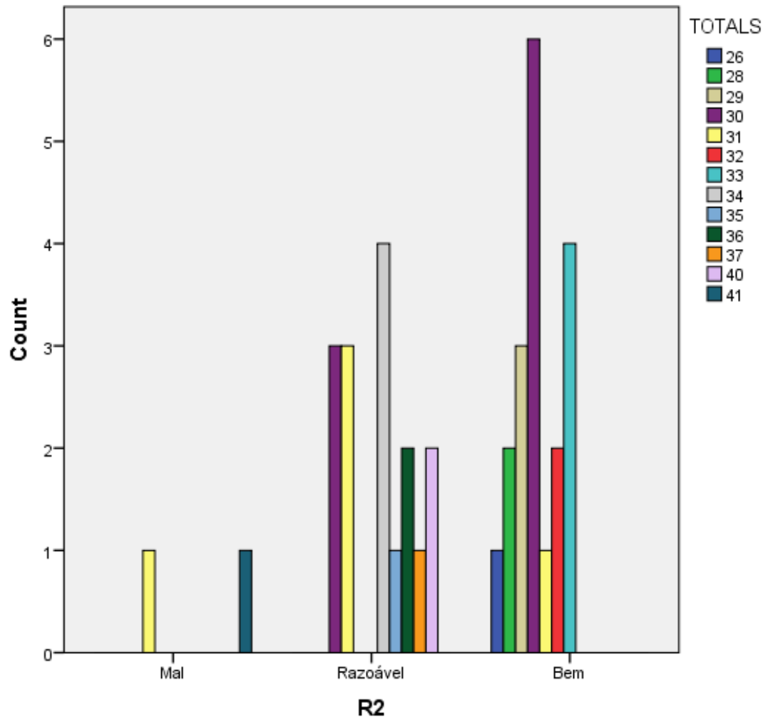
Gráfico 6: Relação entre o R2 e os Totals.
