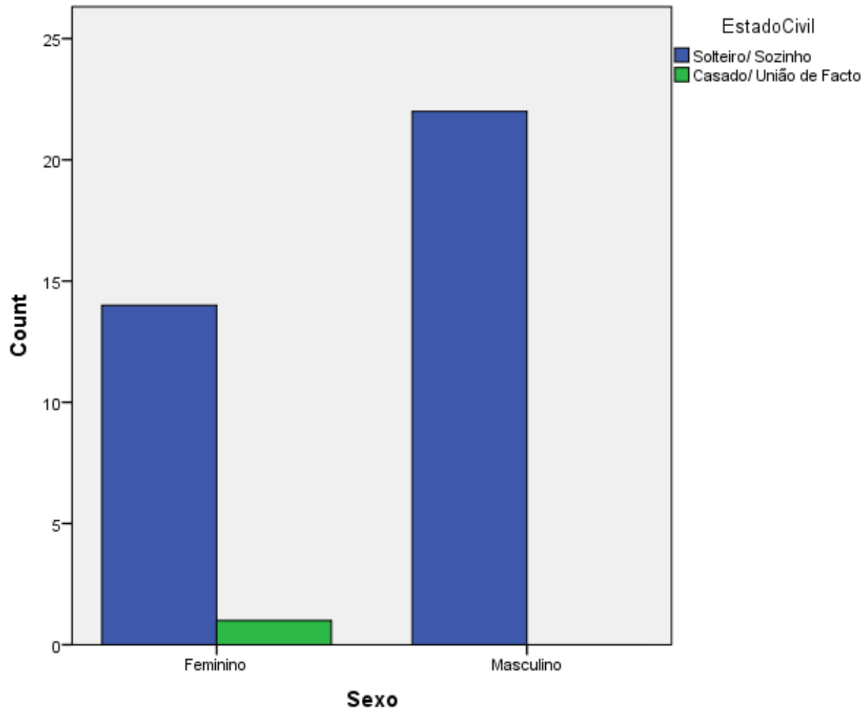
Gráfico 4: Relação entre o Sexo e o Estado Civil.
