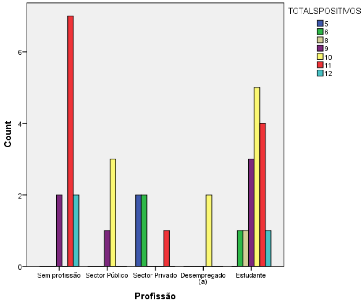
Gráfico 5: Relação entre a profissão e o TotalS positivos.
