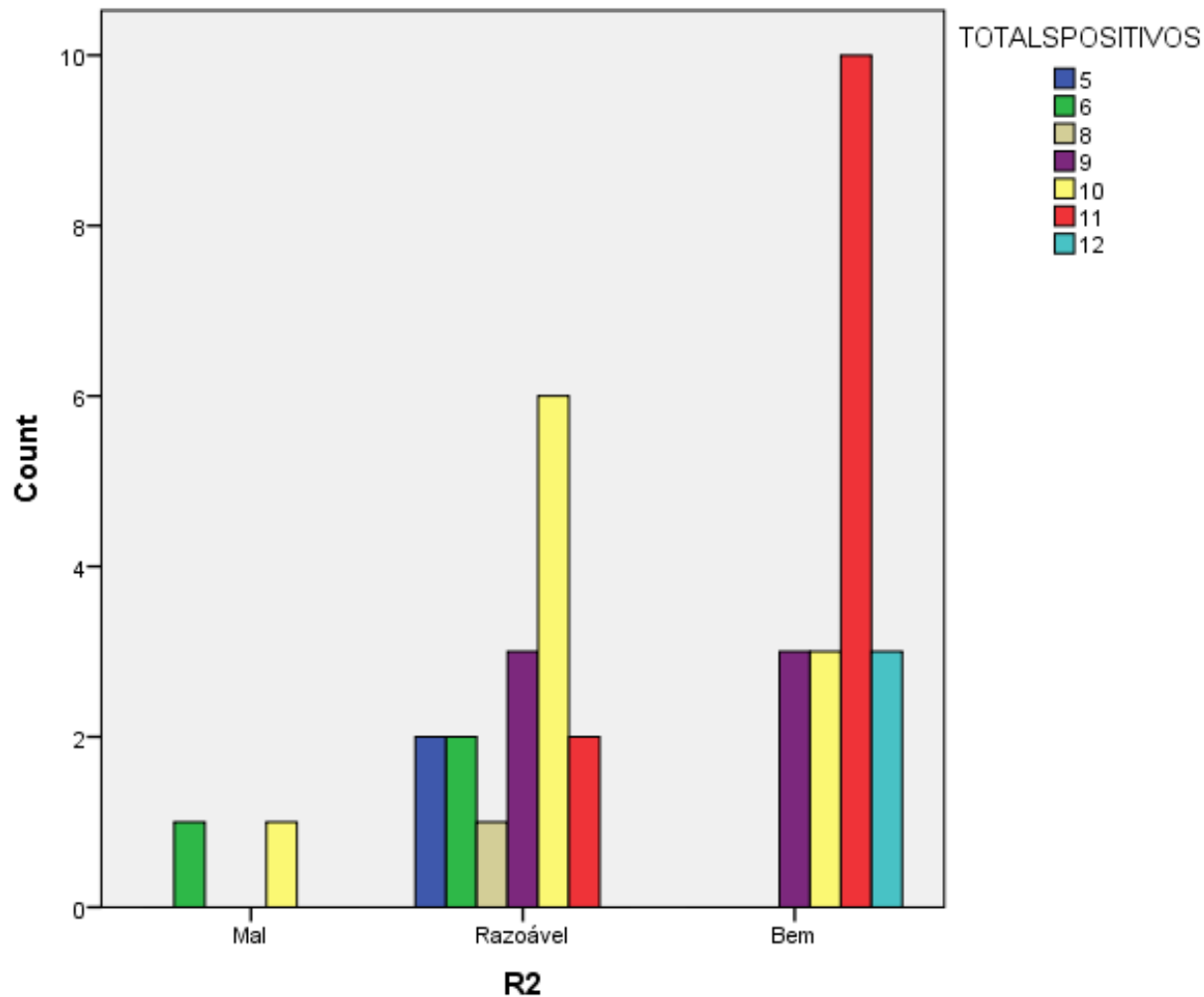
Gráfico 5: Relação entre R2 e o TotalS positivos
